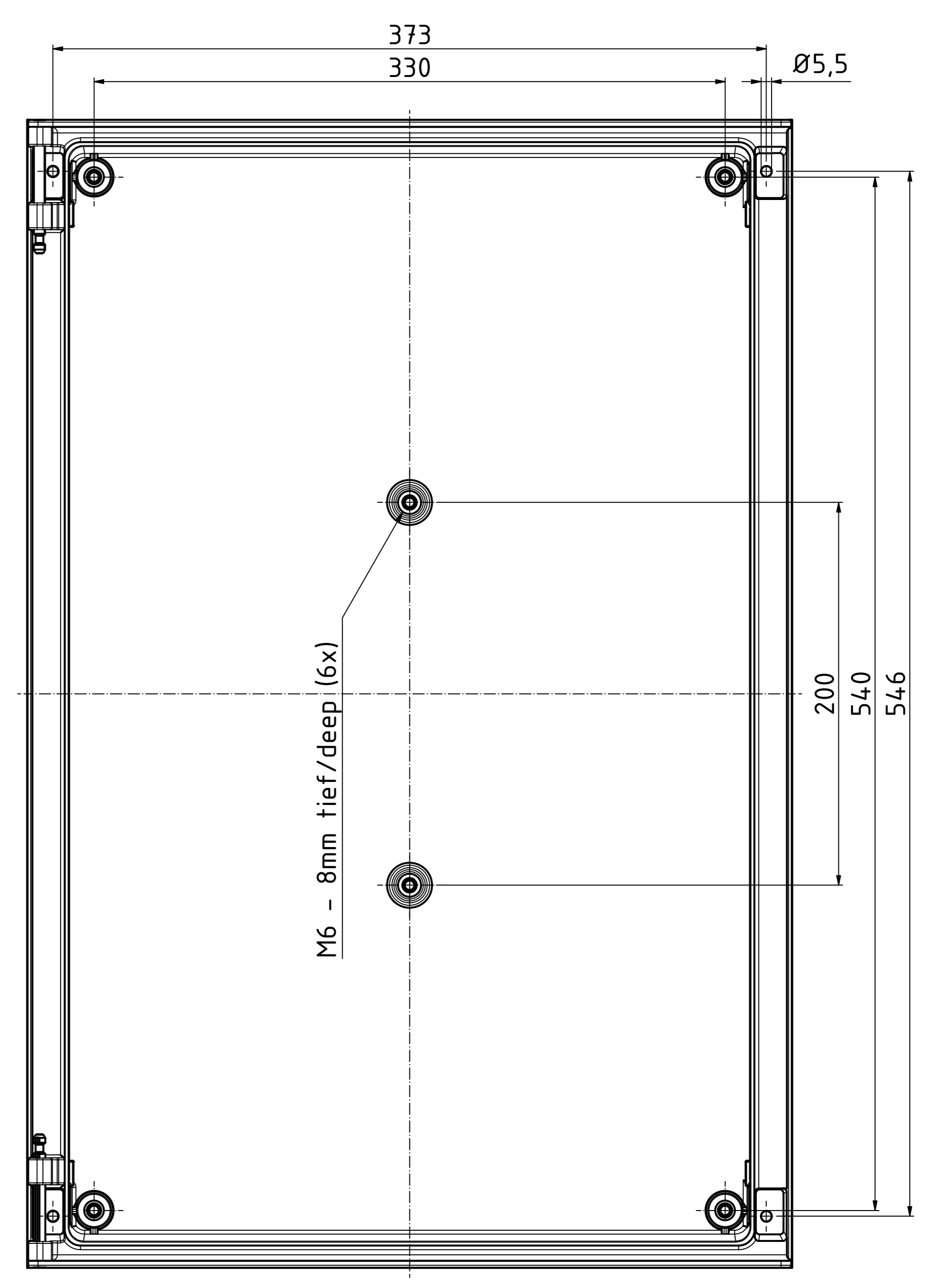
Unterteil ( 1 : 2 ) Base
