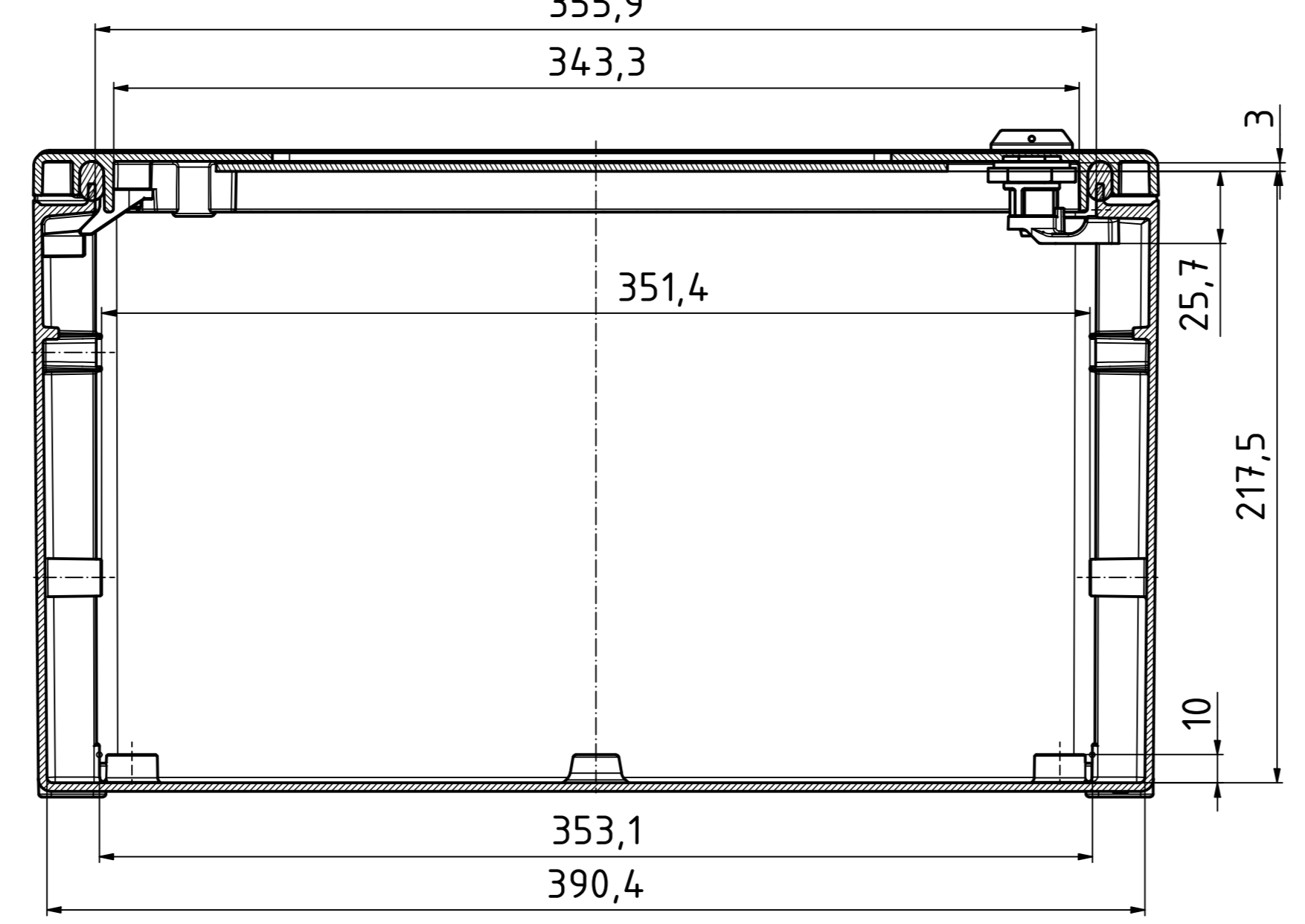
A-A ( 1 : 2 )
