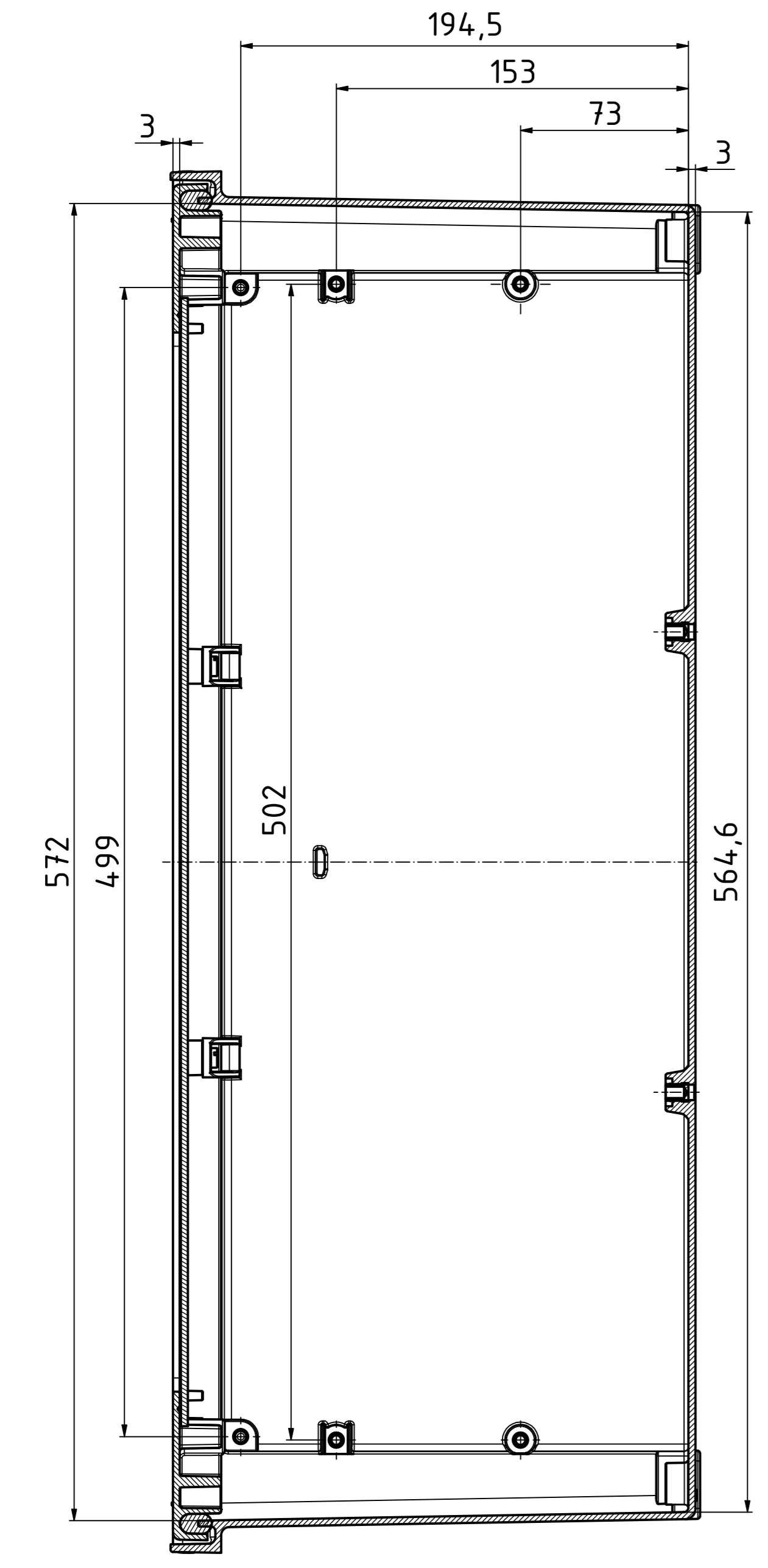
B-B ( 1 : 2 )
