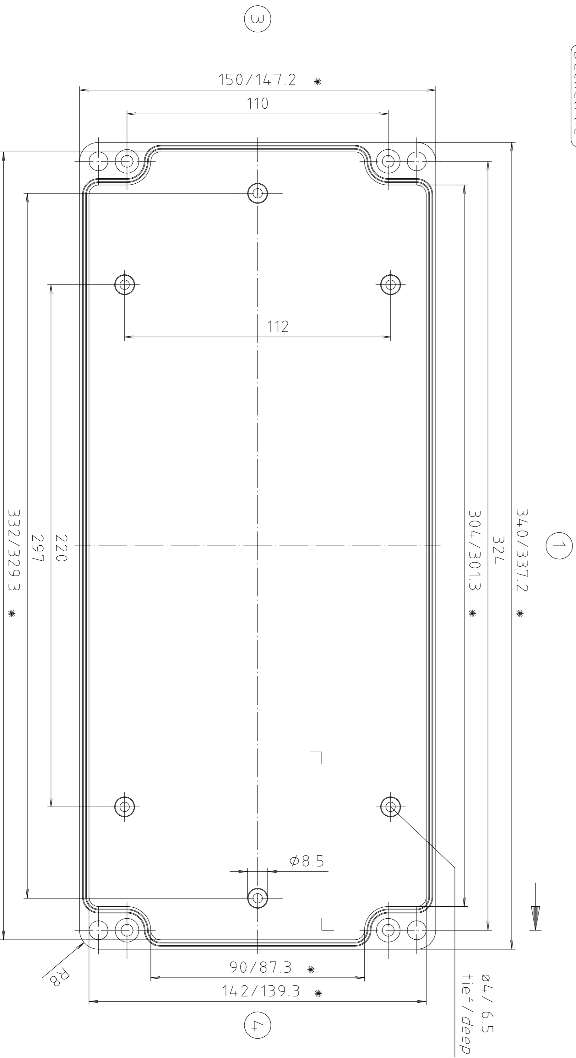
Unterteil/base
