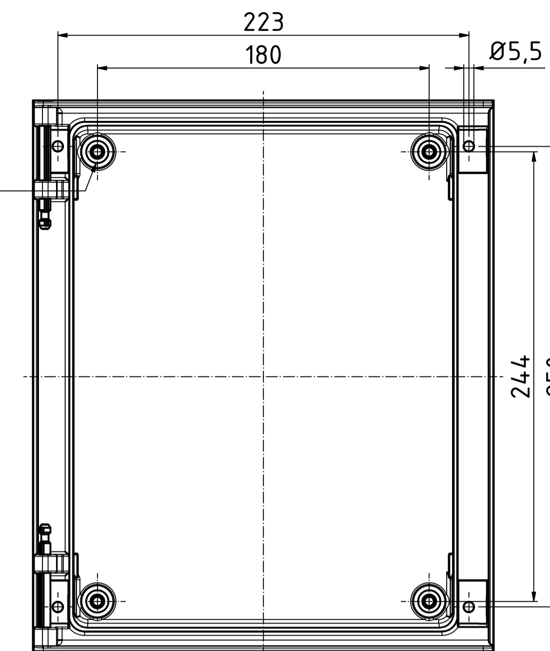
Unterteil/base ( 1 : 2 )
