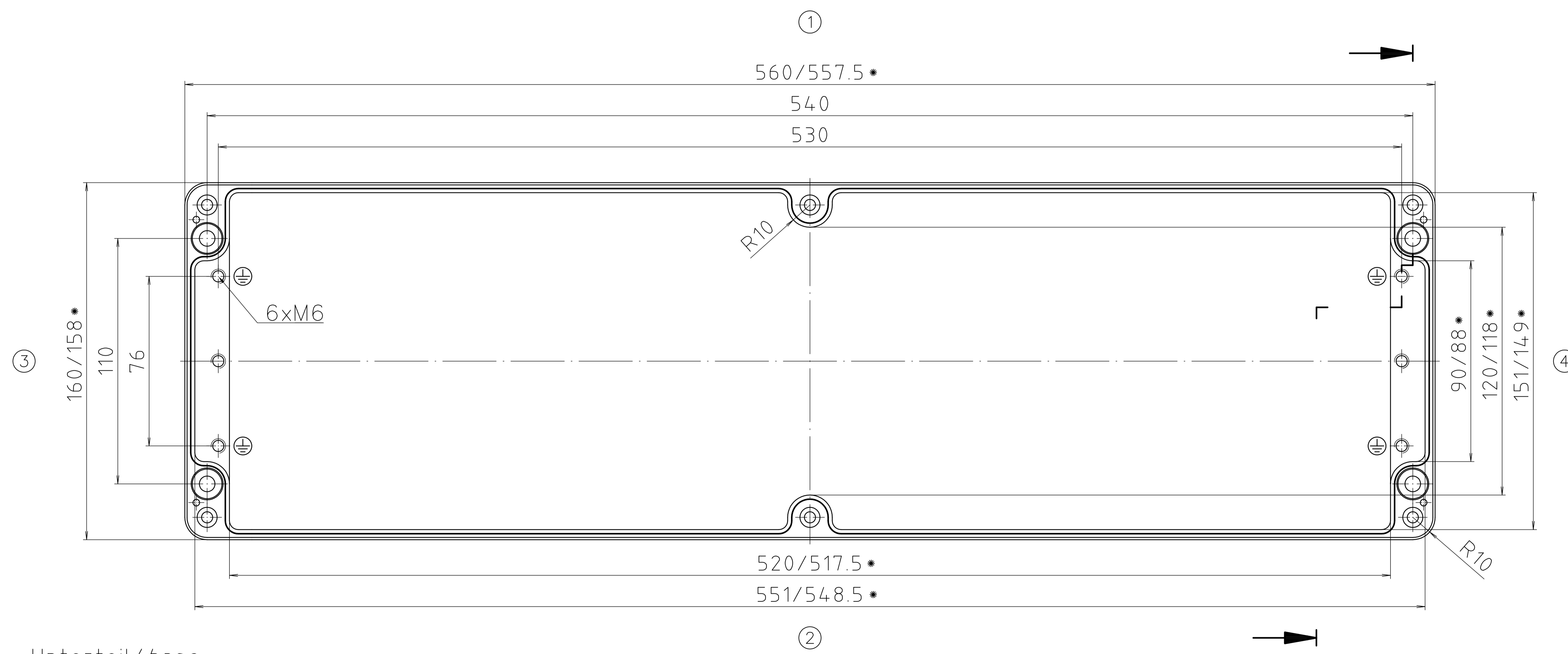
Unterteil / base
