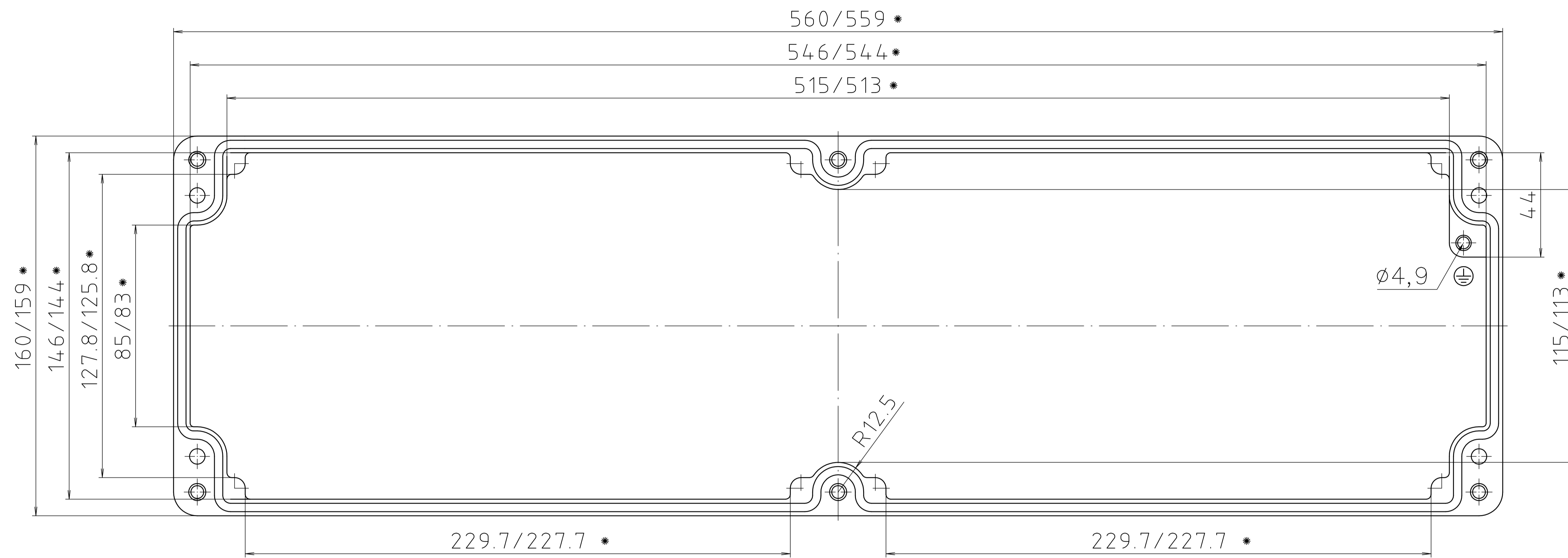
Deckel / lid
