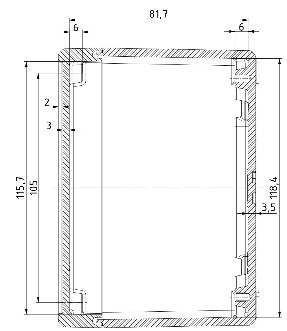
A-A ( 1 : 1 )
