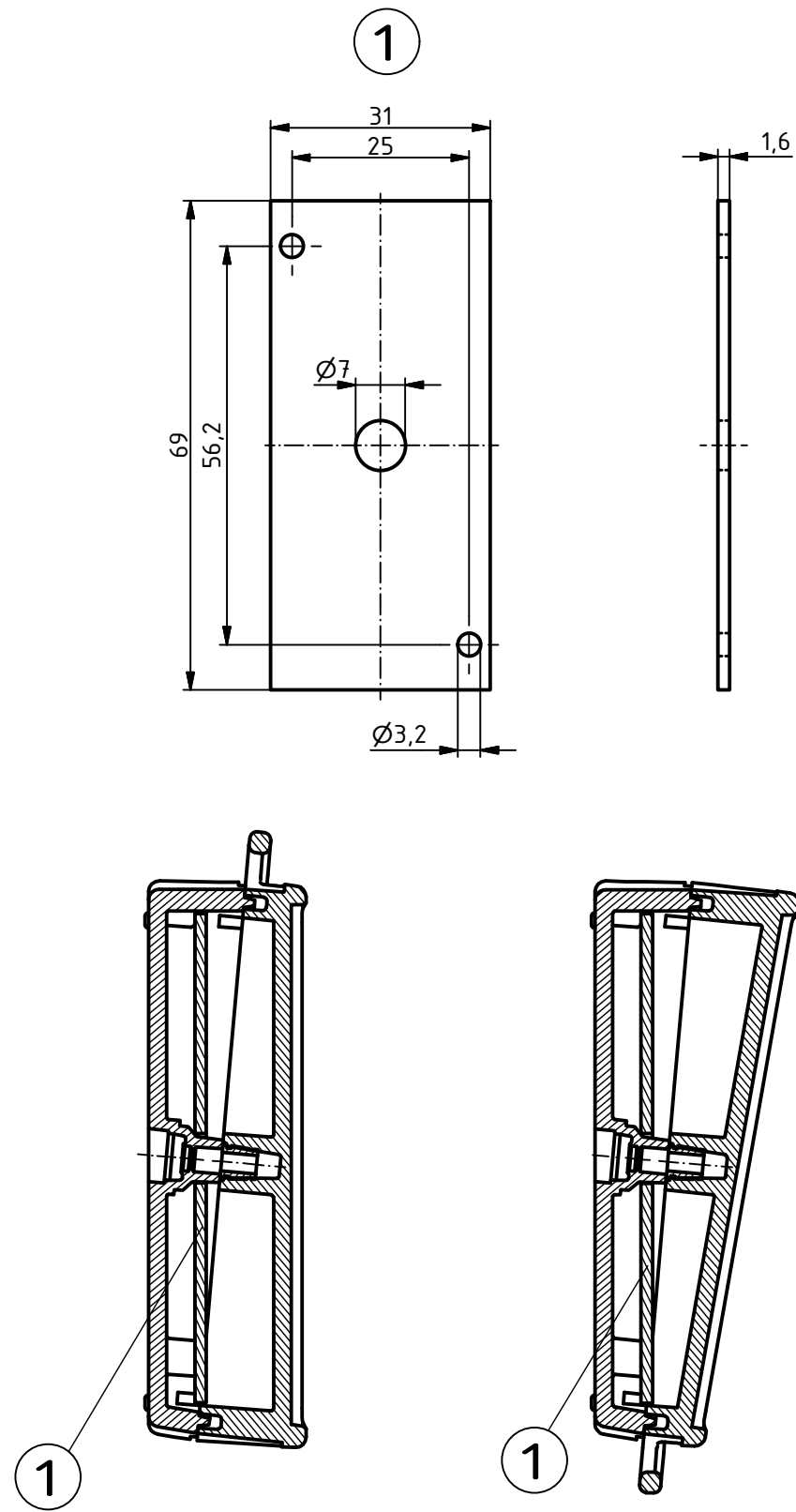
1 BS 200 / 202 (parallel) -Oberteil F -Unterteil BS 200 / 202 (parallel) lid F -base
